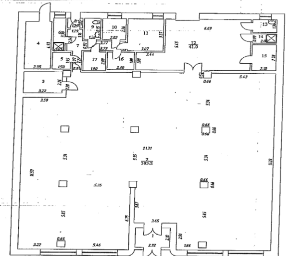
Поэтажный план лит. А - 1 этаж
